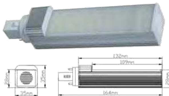
G24-SMD52S
