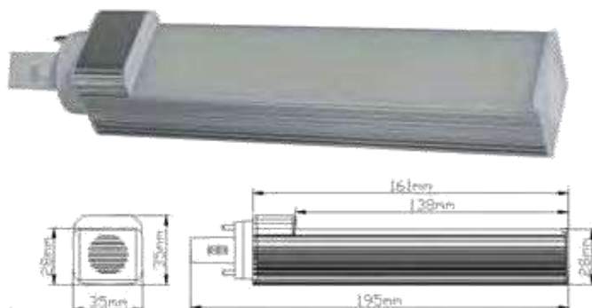
G24-SMD64S
